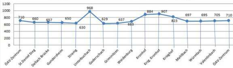
Höhenprofil der Wegstrecke für "MTB-Grenzmarathon" Strecke B Länge ca. 37,5 km - ca. 616 Höhenmeter Anstieg
